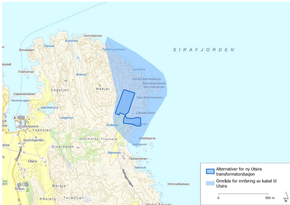
Figur 3. Ilandføringsområde og alternativer for plassering av transformatorstasjon på Utsira meldt av Harald Hårfagre.
