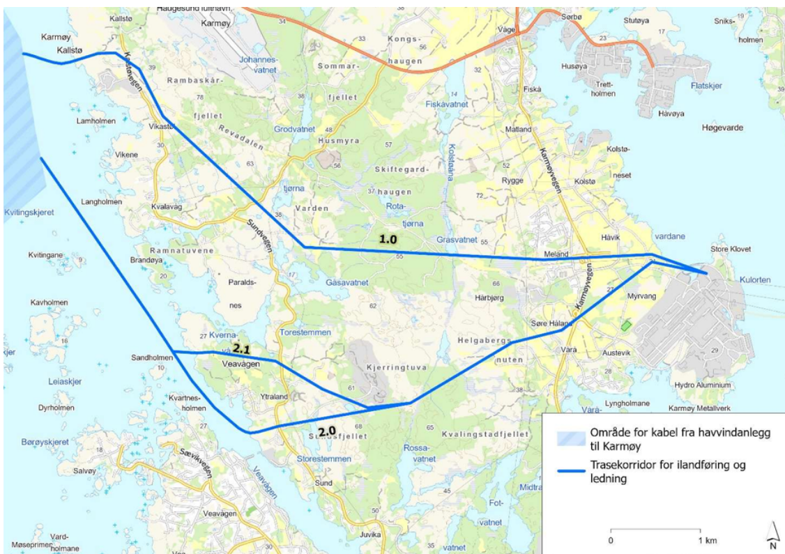
Figur 4. Alternative traseer for luftledning fra landfall vest på Karmøy meldt av Harald Hårfagre til Karmøy transformatorstasjon.
