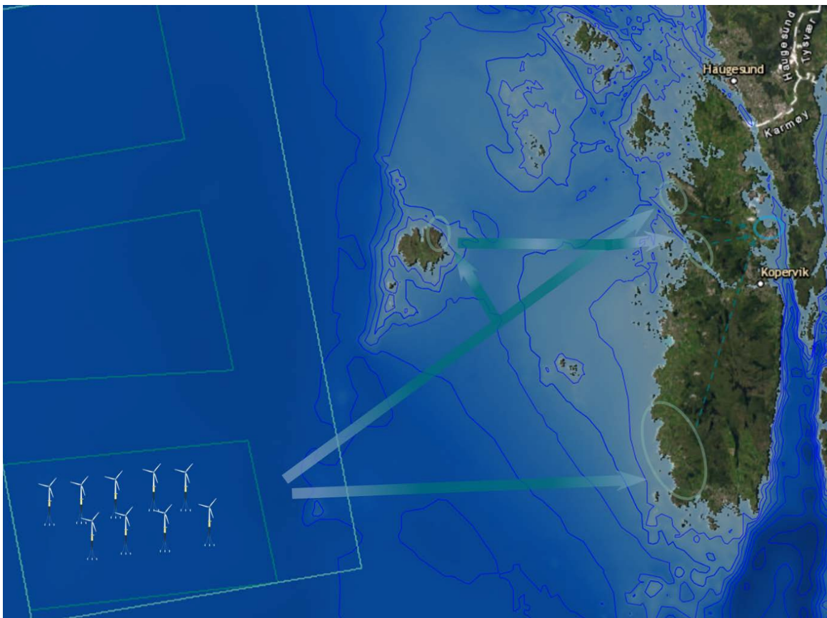
Figur 5. Illustrasjon av lokalisering av havvindanlegget og alternative ruter for sjøkabel meldt av Utsira Nord Havvind.
